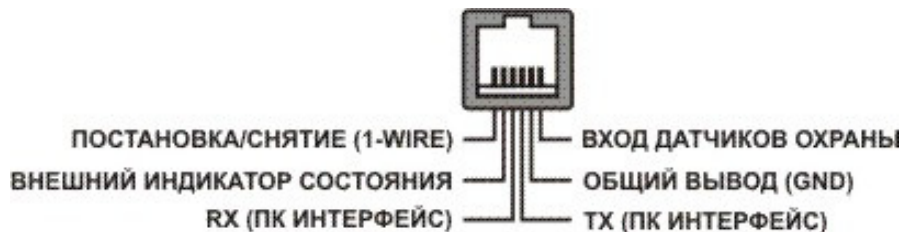
Рисунок 5 – Назначение контактов
