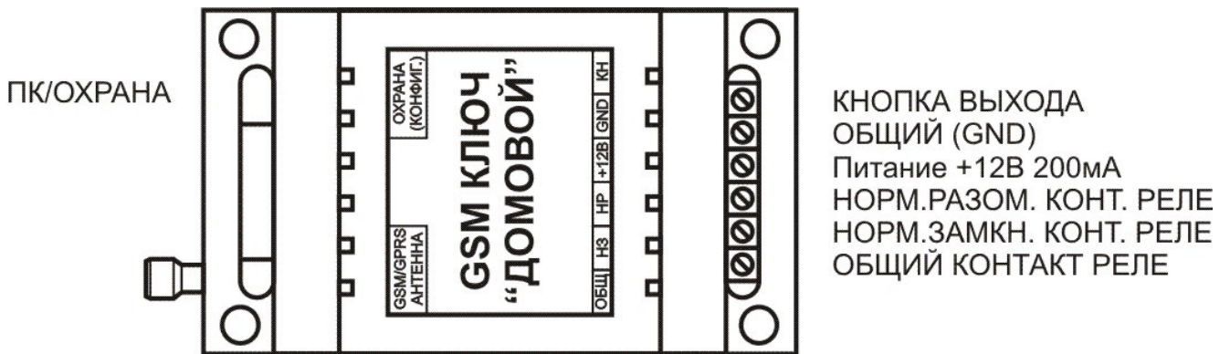
Рисунок 4 – Назначение контактов
